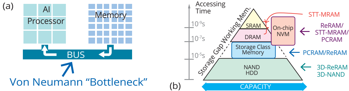
图 4-1 (a) AI 芯片中的冯·诺伊曼“瓶颈” (b) 内存层级结构
