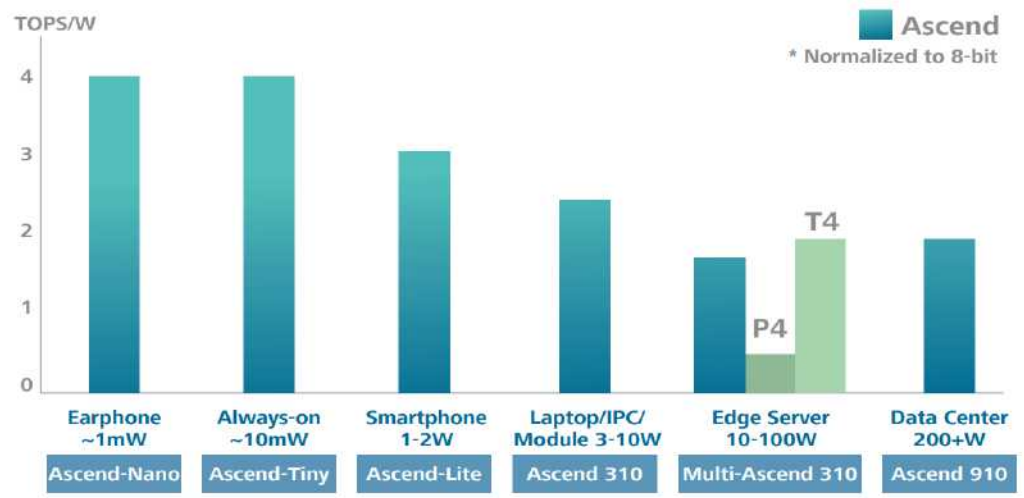
图 2：各类昇腾芯片横跨全场景的最优表现
