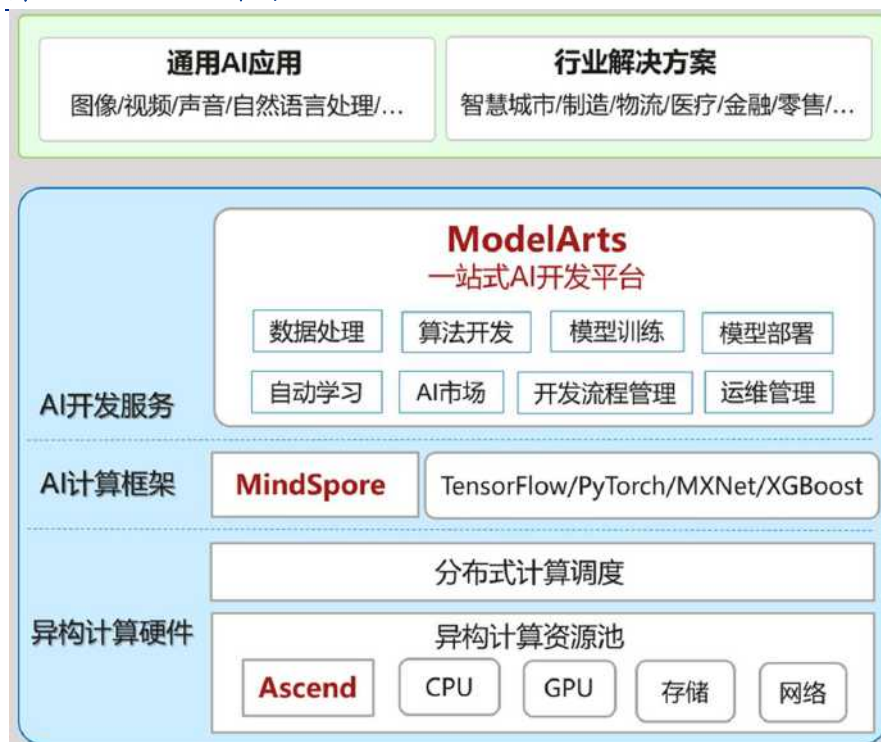
图 22: ModelArts 架构
